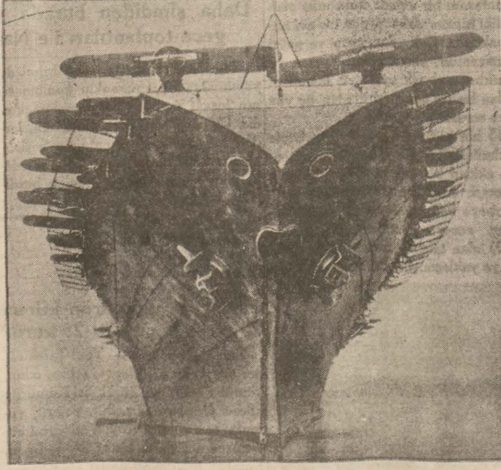
Dünyanın en büyük tayyare gemilerinden Amerikanın (Vatoga) tayyare nakliyesi
